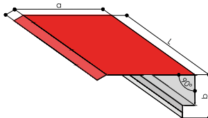
CORONACIÓN EN LATERAL DE PENDIENTE CUBIGREC ROC
