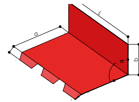
UNIÓN DE FACHADA A ALTO DE PENDIENTE CUBIGREC ROC
